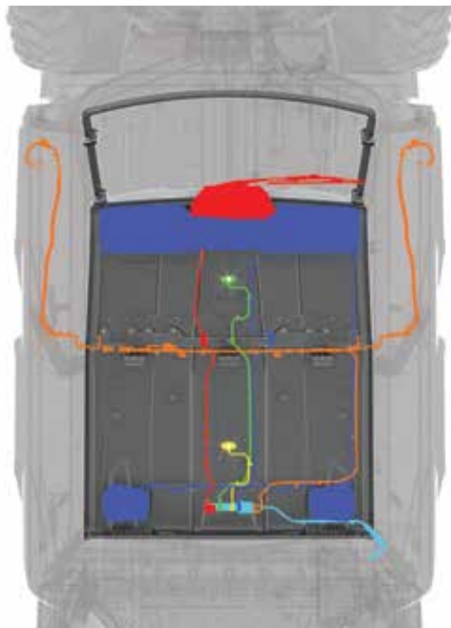
НА РИСУНКЕ ПОКАЗАНА СХЕМА ЭЛЕКТРОПРОВОДКИ POLARIS PULSE В МОДЕЛИ CREW XP 1000
